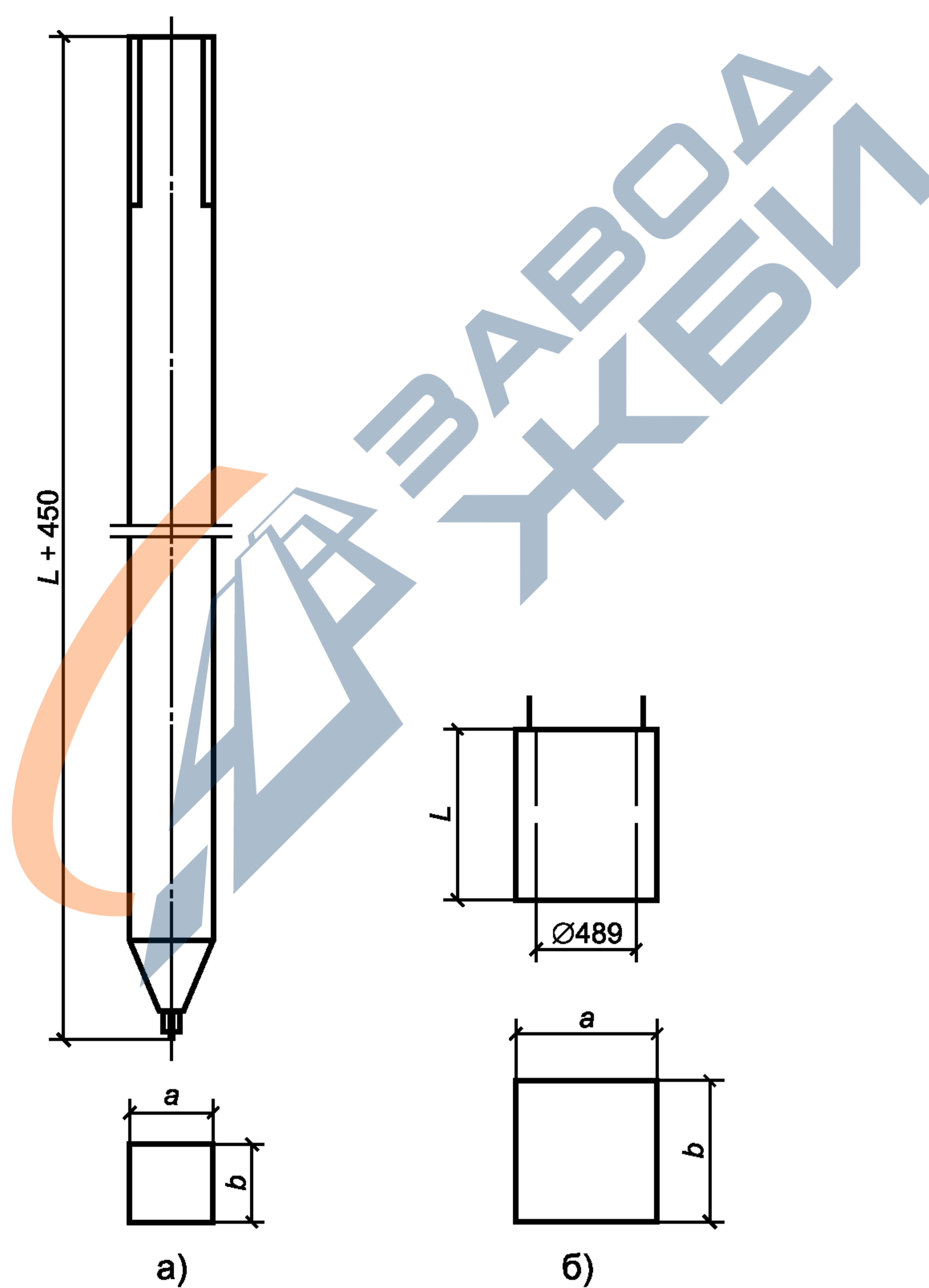
Рисунок 3 — Свая железобетонная с оголовком: а) свая; б) оголовок свайный
